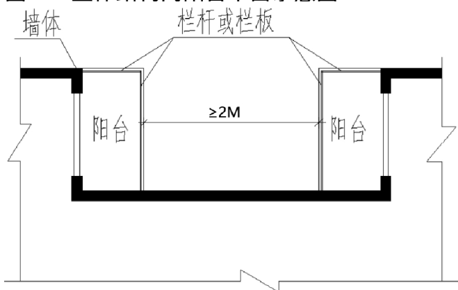
图二：主体结构内阳台平面示意图
