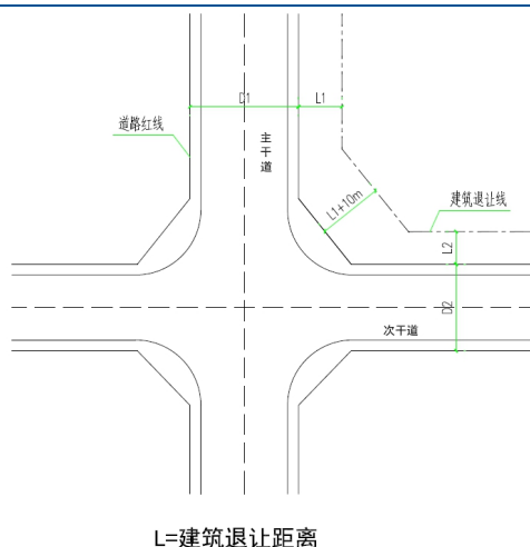
图 5-1 建筑退让计算示意图
