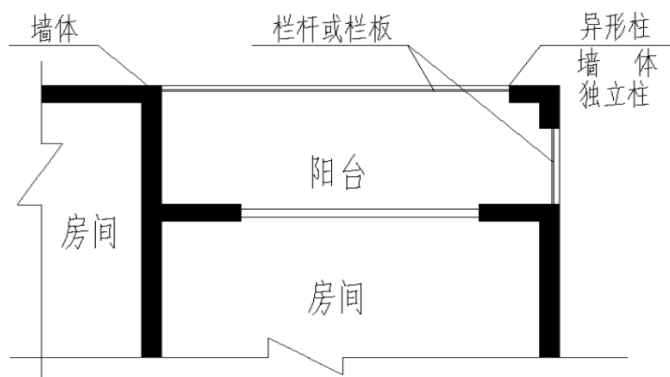
阳台面积计算示意图
